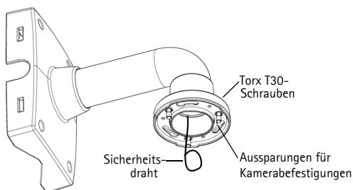
Wandhalterung (Montagebeispiel, Halterung nicht enthalten)
