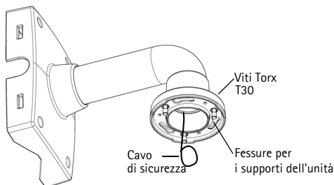
Staffa di montaggio a muro (esempio di montaggio, la staffa non è inclusa)
