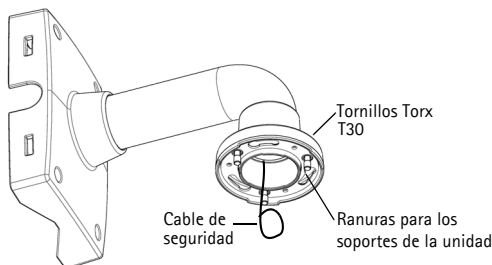
Soporte de pared (ejemplo de montaje, soporte no incluido)
