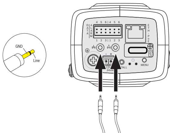
Afbeelding 5.6 Audio-aansluitingen
