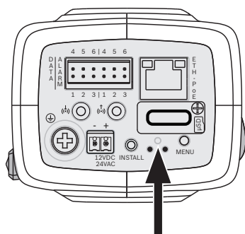
Afbeelding 7.1 Resetknop
