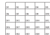
25-split mode
