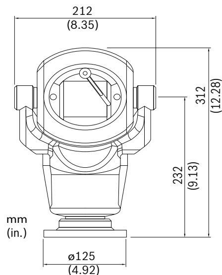
Vooraanzicht, 45° (gekanteld)
