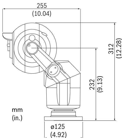
Zijaanzicht, 45° (gekanteld)
