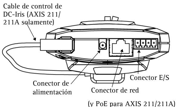
Panel posterior AXIS 210/211
