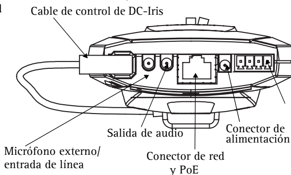
Panel posterior AXIS 211A
