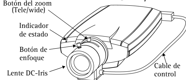
Botón del zoom (Tele/wide) AXIS 211/211A
